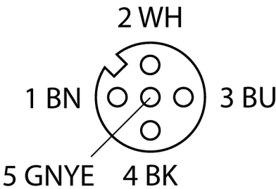
schéma de connexions
