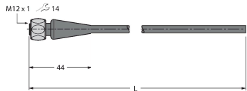
Dibujo acotado Tipo N.º de ID
