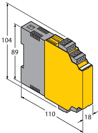
Dibujo acotado Tipo N.º de ID IM72-11EX/L 7520703 conexión de bornes roscada
