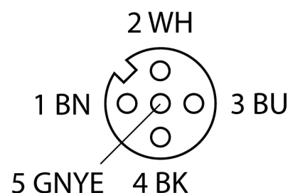
Schéma zapojení
