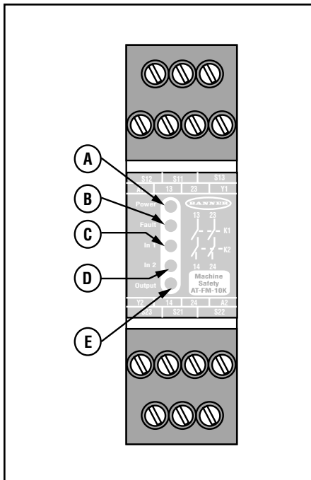
Abb. 1 LED-Anzeigen und Klemmenanordnung am DUO-TOUCH SG Sicherheitsmodul AT-FM-10K
