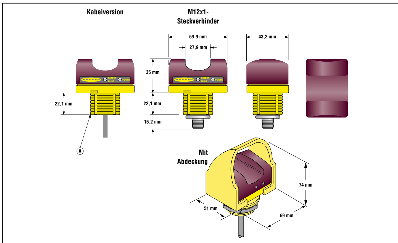
Abb. 7 Abmessungen der STB-Taster
