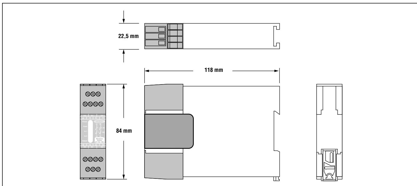
Abb. 6 Abmessungen des DUO-TOUCH SG Sicherheitsmoduls
