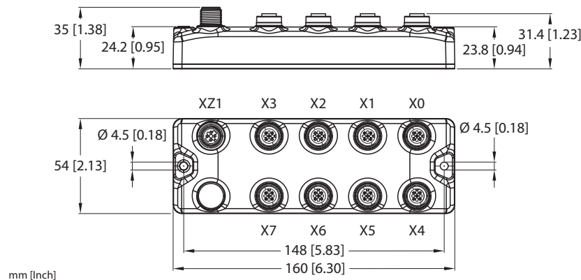
Fig. 1: Dimensions
